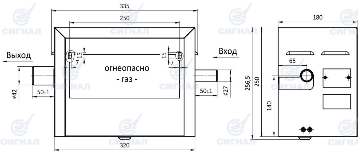
Рисунок 7 - Габаритно-установочная схема пункта ГРПШ-10-1-ПЛ-М; ГРПШ-10М-1-ПЛ-М
