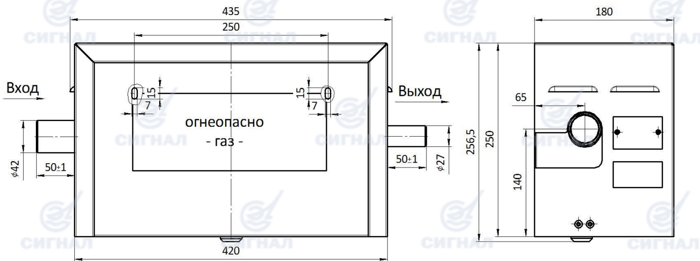
Рисунок 11 – Габаритно-установочная схема Пункта ГРПШ-10М-1-ПЛ-ПП; ГРПШ-10-1-ПЛ-ПП; ГРПШ-10М-1-ПЛ-ММ; ГРПШ-10-1-ПЛ-ММ
