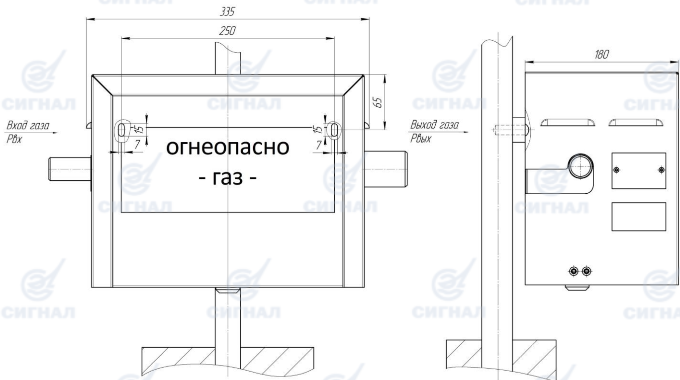
Рисунок 7 - Габаритно-установочная схема пункта ГРПШ-10-1-ПЛ-М; ГРПШ-10М-1-ПЛ-М
