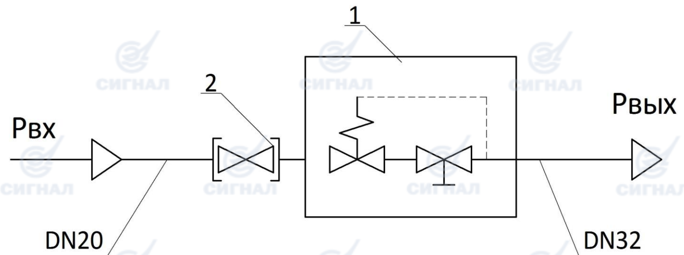
1 - Регулятор, 2- кран DN20(кран под приварку или муфтовый, в зависимости от исполнения) Рисунок 2.
