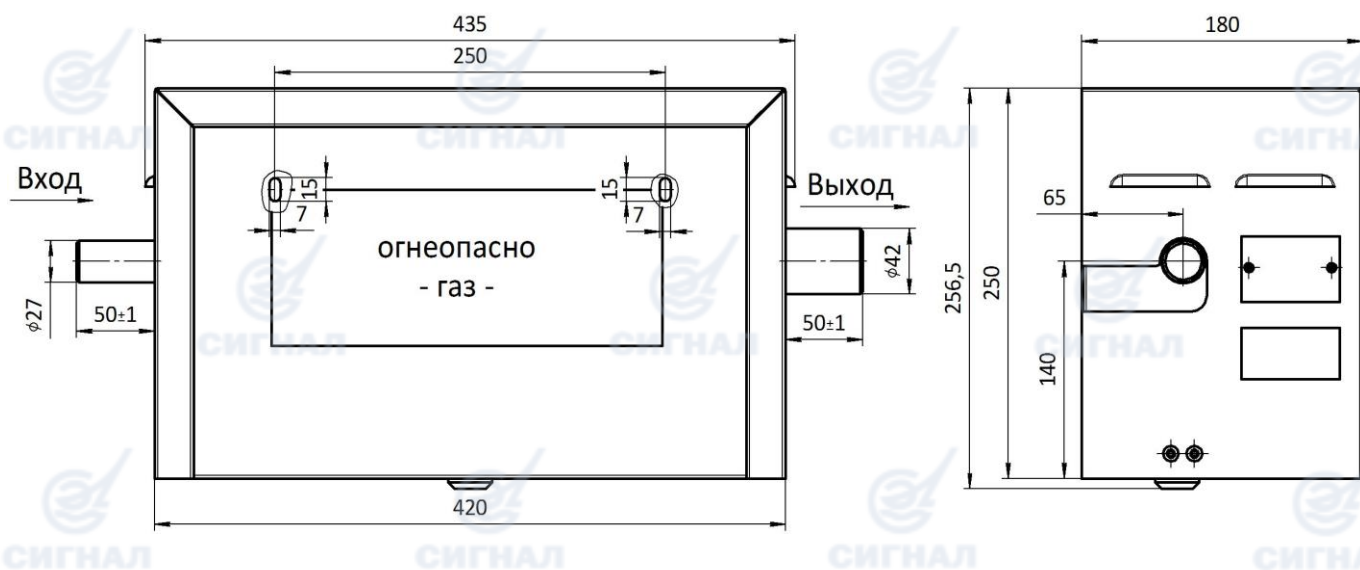
Рисунок 6 - Габаритно-установочная схема пункта ГРПШ-10М-1-ЛП-ПП; ГРПШ-10-1-ЛП-ПП; ГРПШ-10М-1-ЛП-ММ; ГРПШ-10-1-ЛП-ММ.
