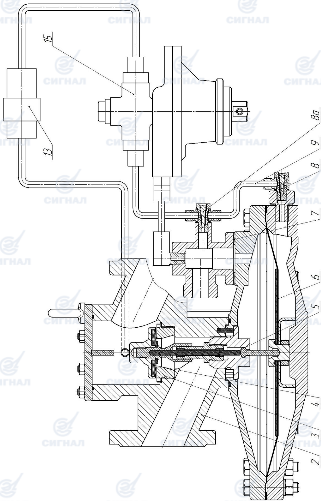
2-исполнительное устройство; 3-седло; 4-клапан рабочий; 5-стержень; 6-мембрана исполнительного устройства; 7-дроссельная шайба; 8, 8а-дроссели регулируемые; 9-грубка импульсная входного газопровода; 10-пружина отсечного клапана; 13-фильтр; 15-регулятор управления (КВ-2);
