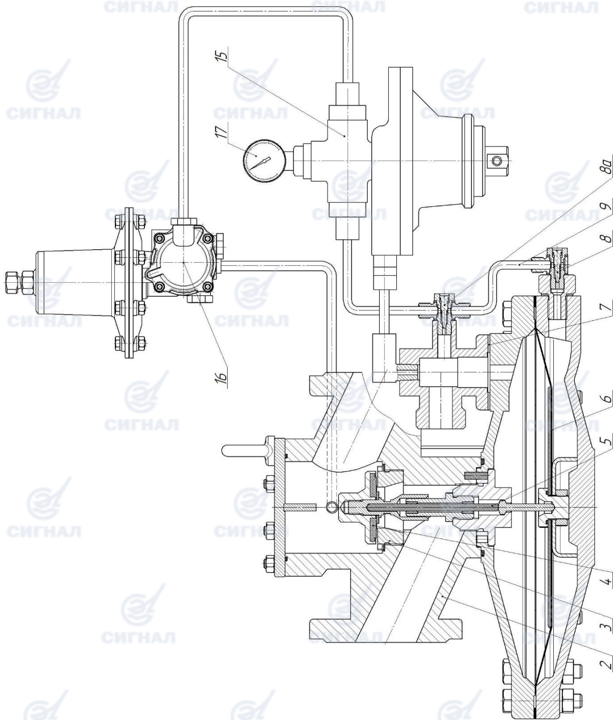
2-исполнительное устройство; 3-седло; 4-клапан рабочий; 5-стержень; 6-мембрана исполнительного устройства; 7-дрессельная шайба; 8-дрессели регулируемые; 9-трубка импульсная входного газопровода; 15-регулятор управления (КН-2); 16-стабилизатор; 17-манометр;
