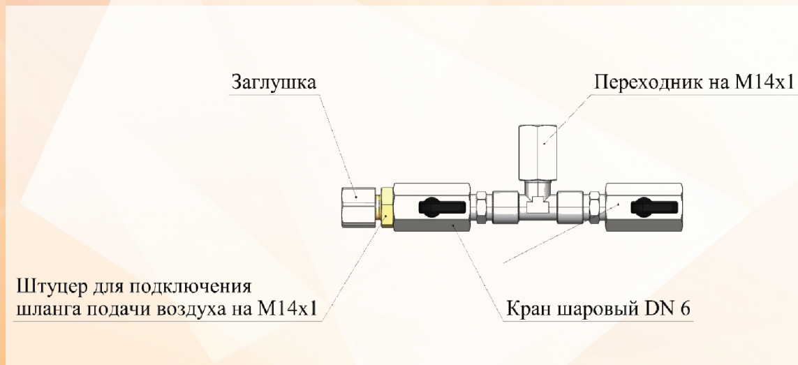
Рисунок 1. Устройство настройки узла ПЗК
