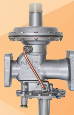
РДСК-50М
