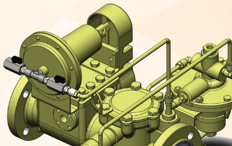
Рисунок 4. Пример монтажа Устройства на регулятор РДГ-2
