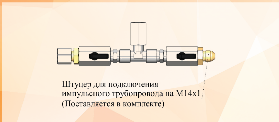
Рисунок 2. Устройство настройки узла ПЗК для регуляторов РДГ (до 2015г.)
