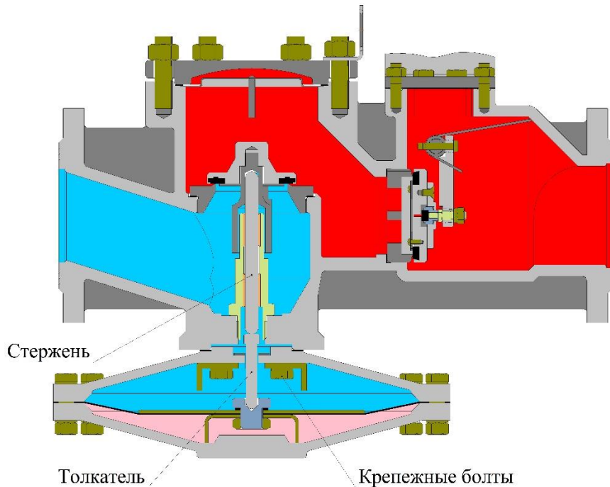
Исполнительное устройство в регуляторах РДГ-2
