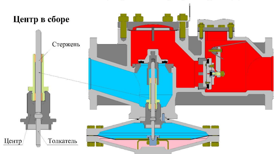
Исполнительное устройство в регуляторах РДГ-3
