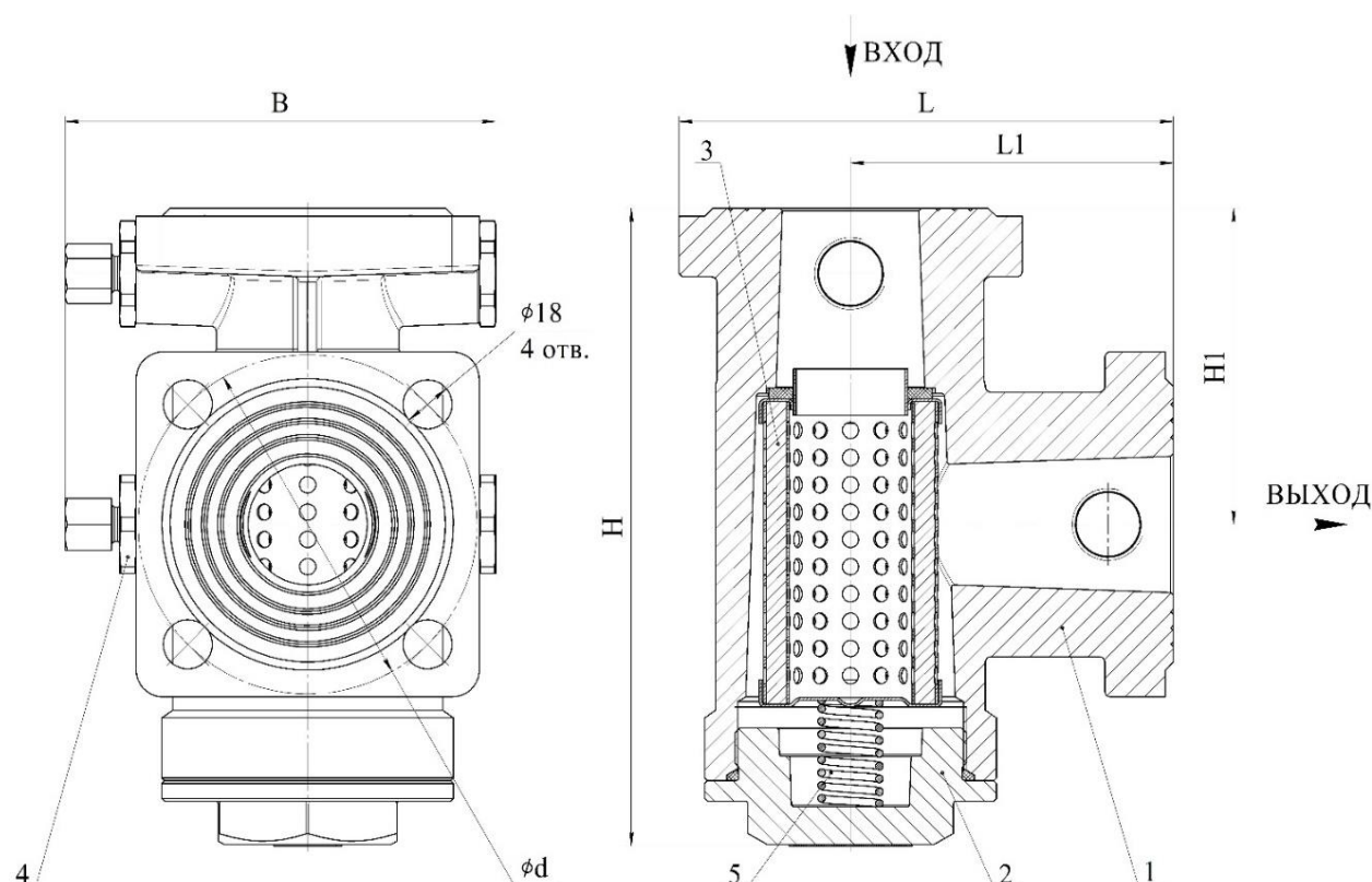
Рисунок 2 – Устройство фильтра ФГ-2
