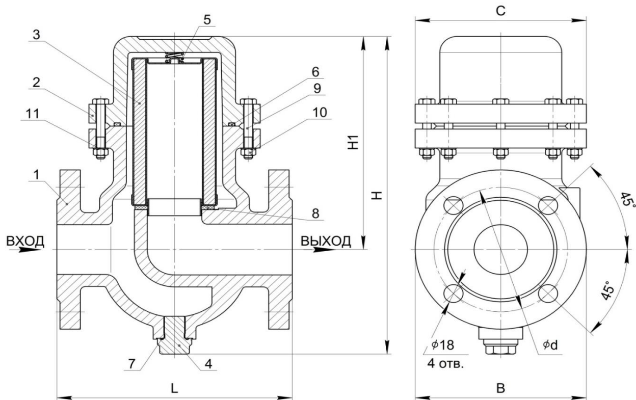
Рисунок 1 – Устройство фильтра ФГ
