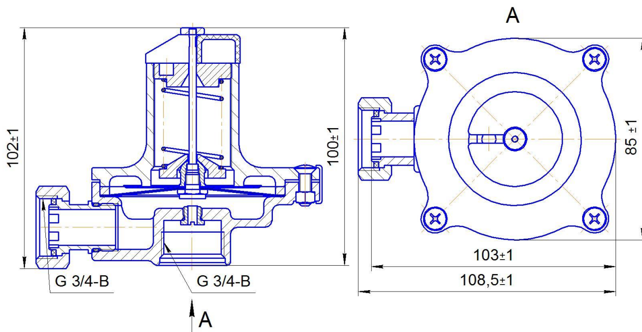
Рисунок 4 – Габаритная схема клапанов КПС-Н-1-Г (С-1-Г; С-2-Г)
