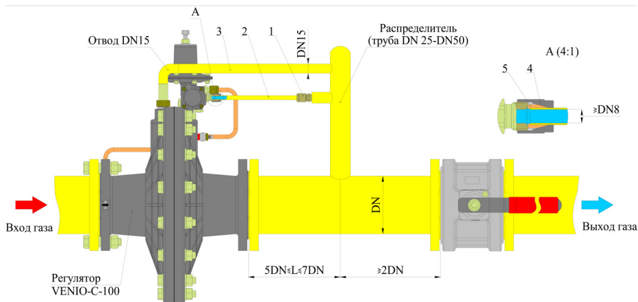
Рисунок 14 - Схема подключения импульсных трубопроводов к регуляторам VENIO-C-100
