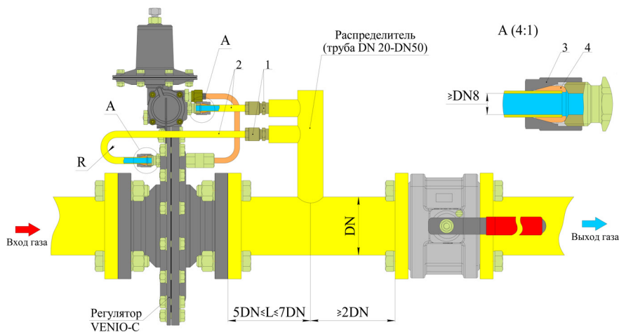
Рисунок 13 - Схема подключения импульсных трубопроводов к регуляторам VENIO-C-50 (-80)
