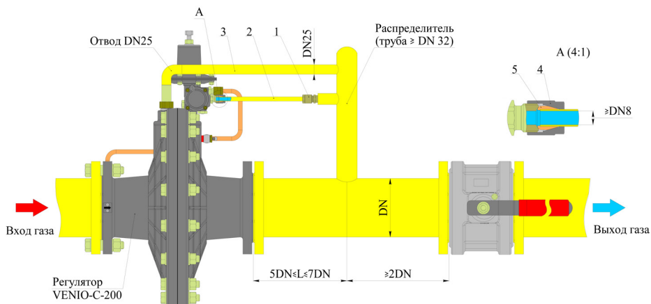
Рисунок 15 - Схема подключения импульсных трубопроводов к регуляторам VENIO-C-200
